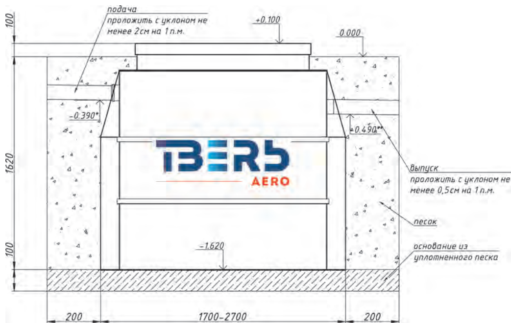
Рисунок 1. TVERЬ АЭРО с самотечным отводом очищенных сточных вод.
