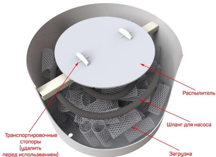
Рисунок 2 – Аэрационный модуль
