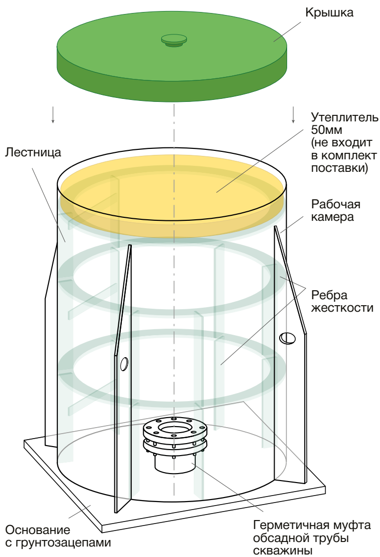
Пластиковый кессон Евролос
