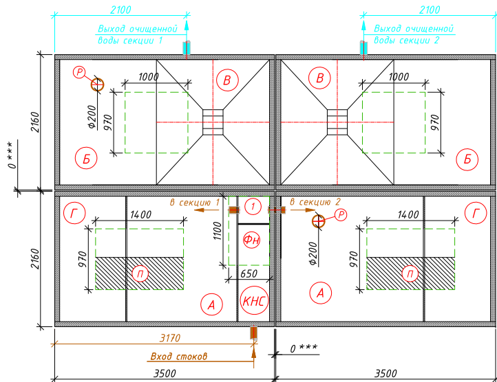
Схема станции
