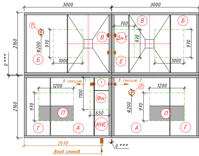
Схема станции
