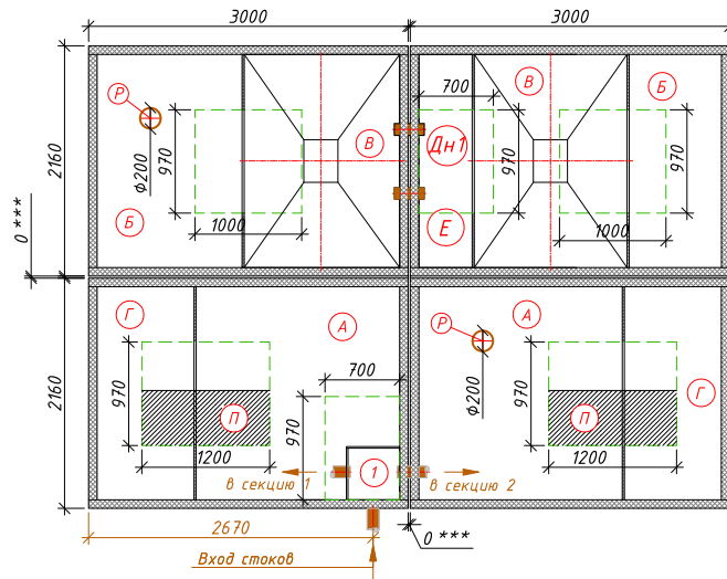
Схема станции
