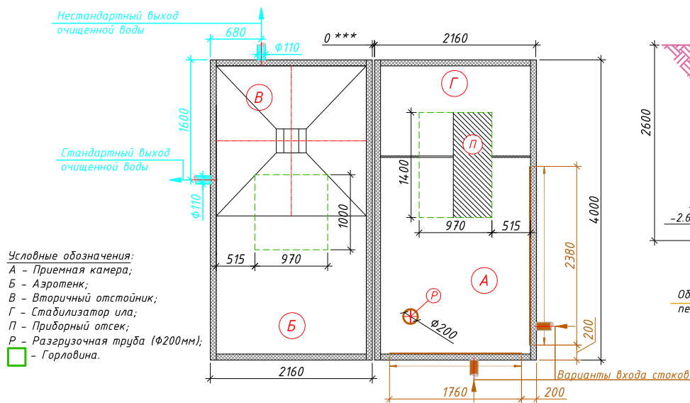
Схема станции
