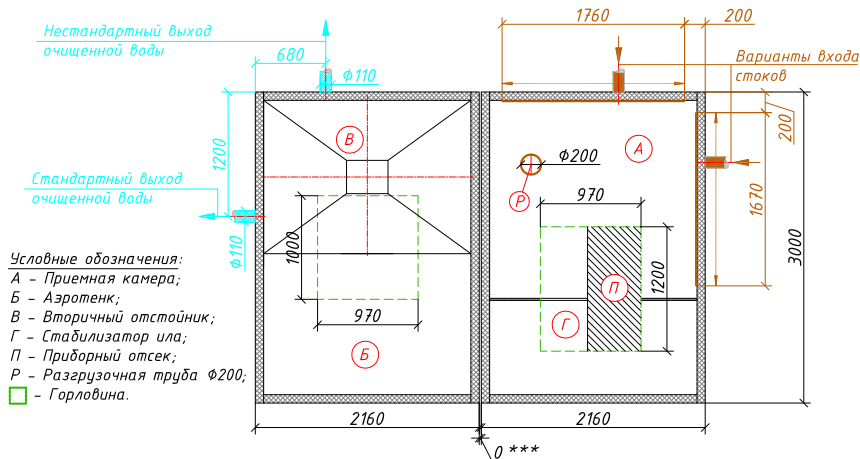
Схема станции
