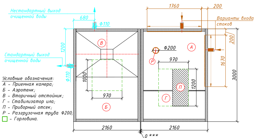
Схема станции
