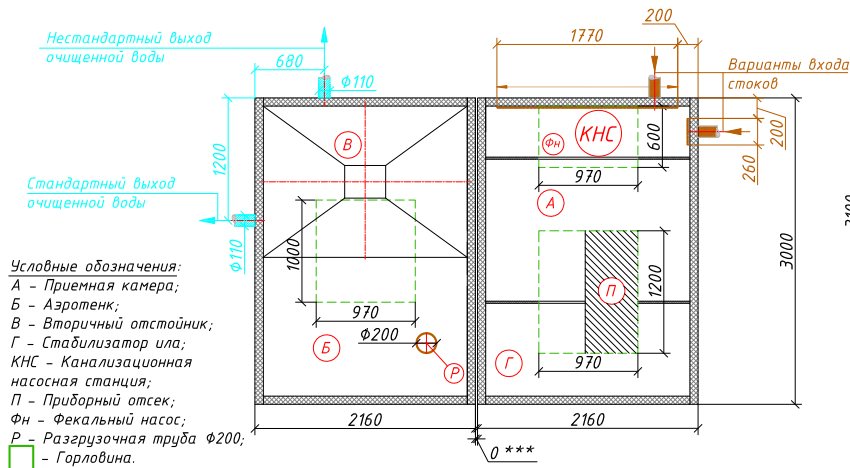
Схема станции
