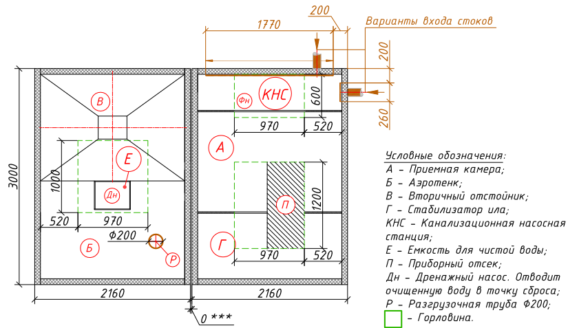
Схема станции
