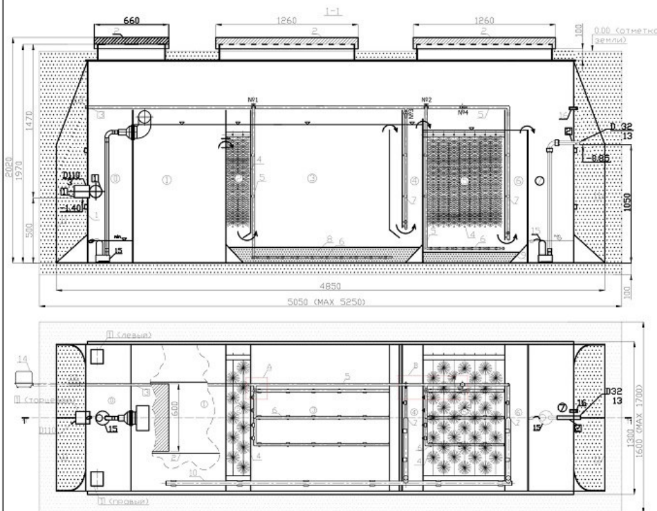
Фрагмент А
